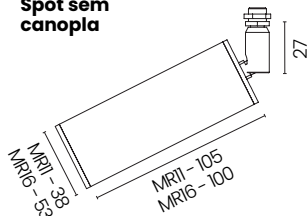
Spot com prolongador e sem canopla
